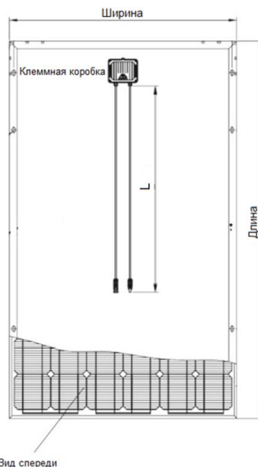
Рисунок 1 – схематическое изображение ФЭМ
